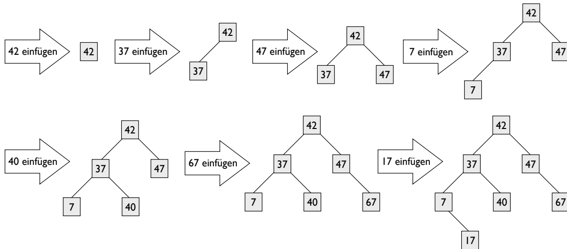
Abbildung 7.1: Beispiel für einen binären Suchbaum
