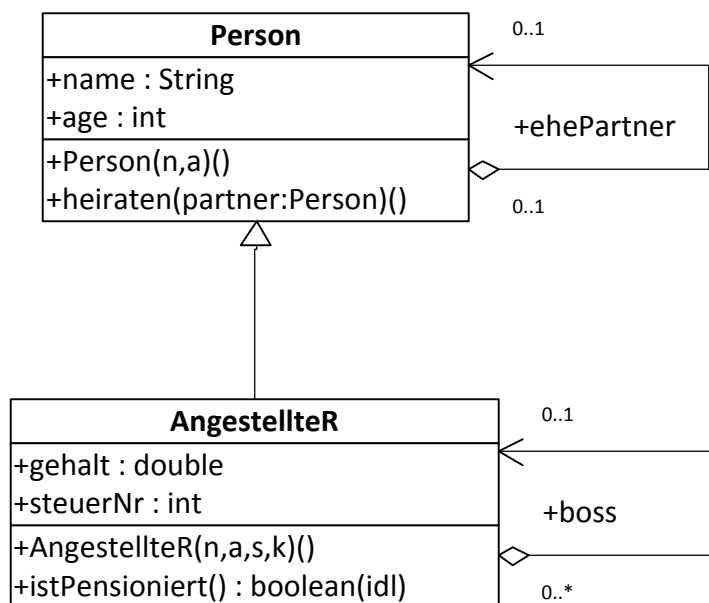
Abbildung 3.2: Die Generalisierung/Spezialisierung
