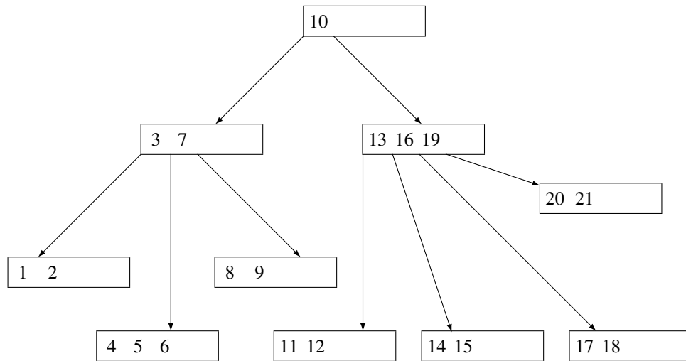
Abbildung 7.13: Einfügen einer 17
