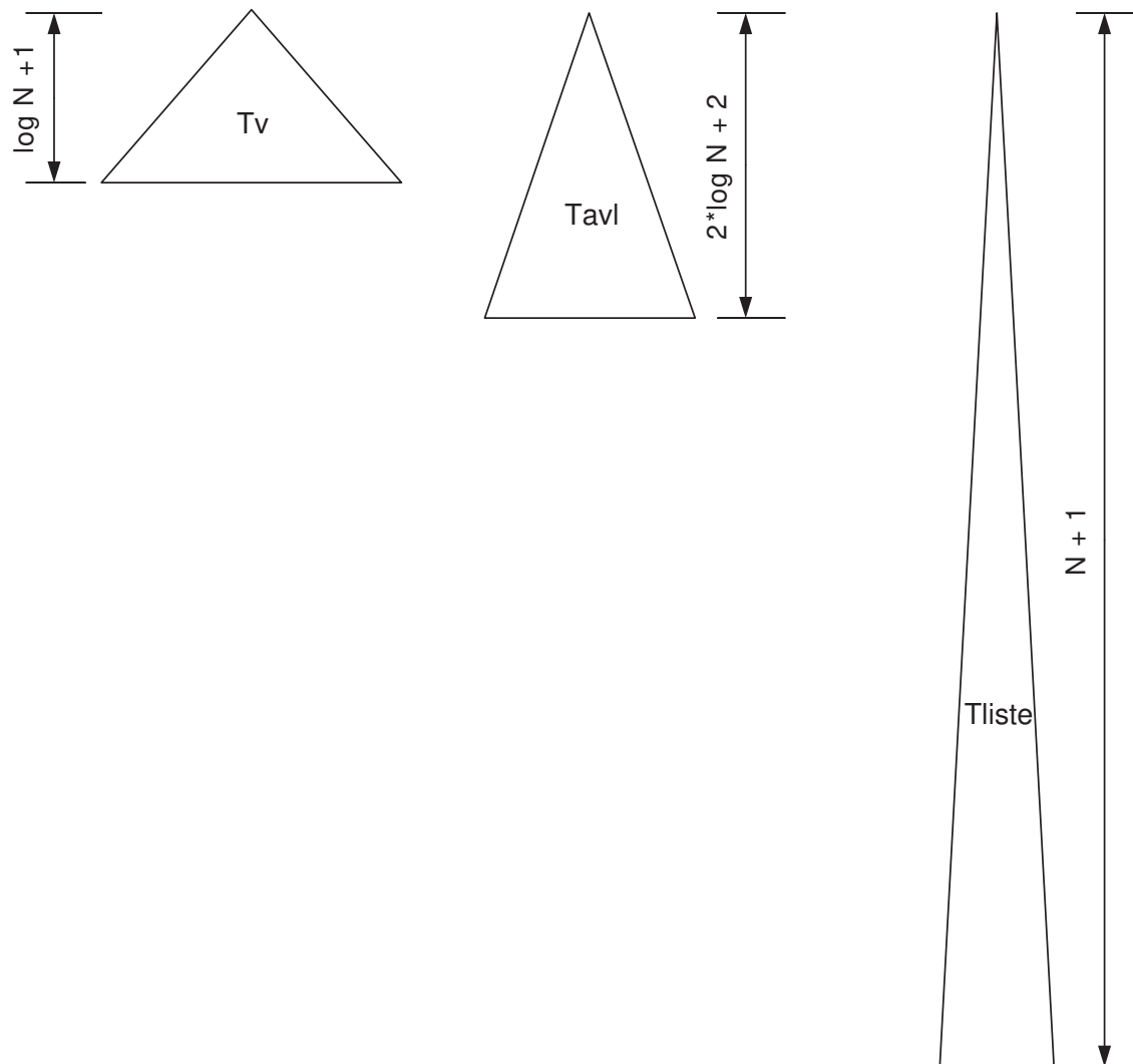
Abbildung 7.4: Höhenvergleich: vollständiger Suchbaum, AVL-Baum, degenerierter Suchbaum
