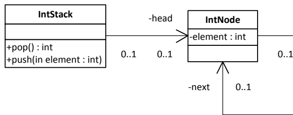
Abbildung 2: Stack mit verketteter Liste
